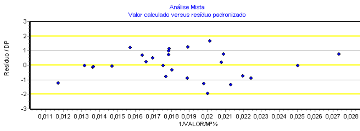
Figura 06 - Gráfico de resíduos.
