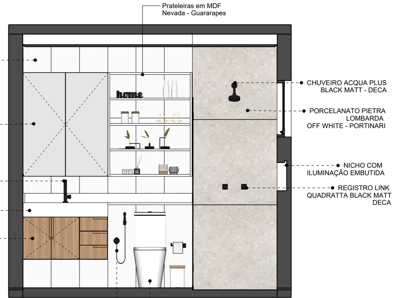
Vista A Humanizada - Banheiro
