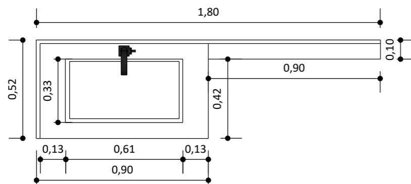
Vista Superior - Bancada
