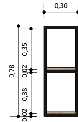
Vista Lateral Direita - Prateleira Suspensa
