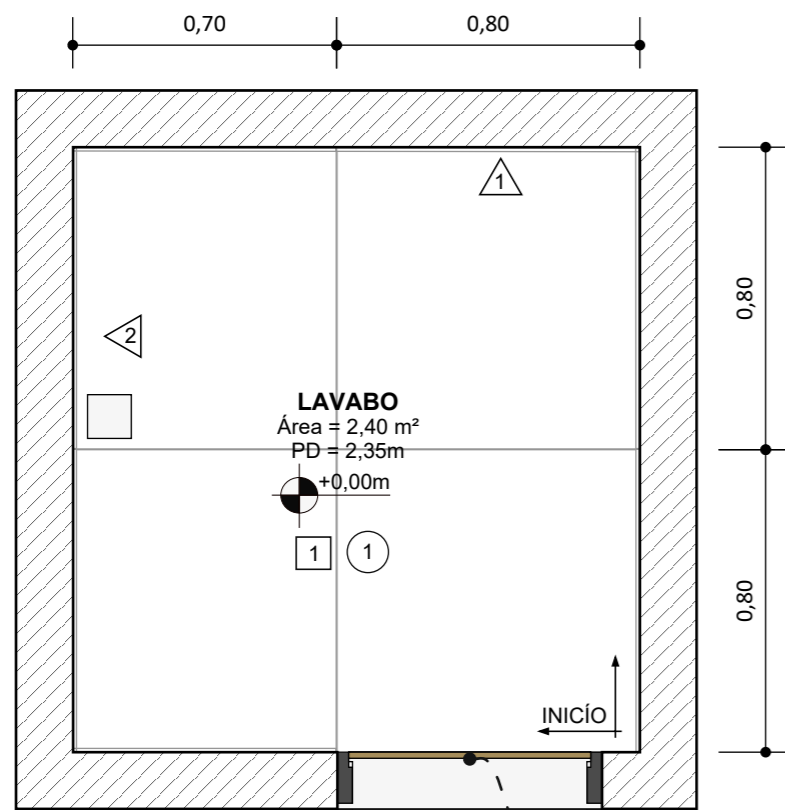
Planta de Paginação
