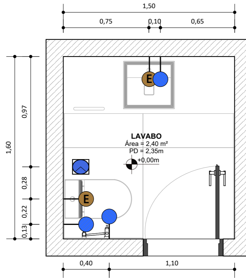
Planta de Pontos Hidráulicos
