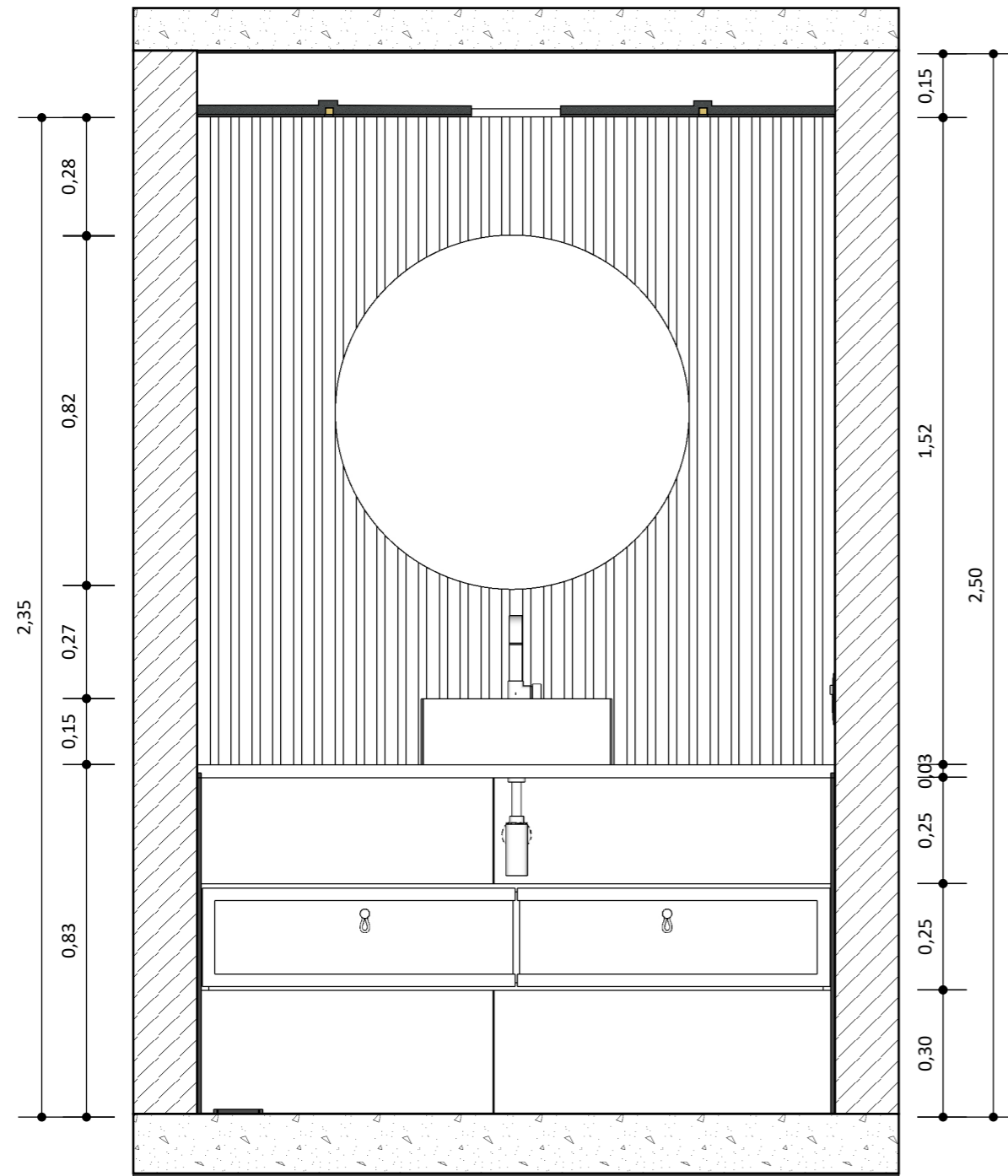
Corte A Técnico
