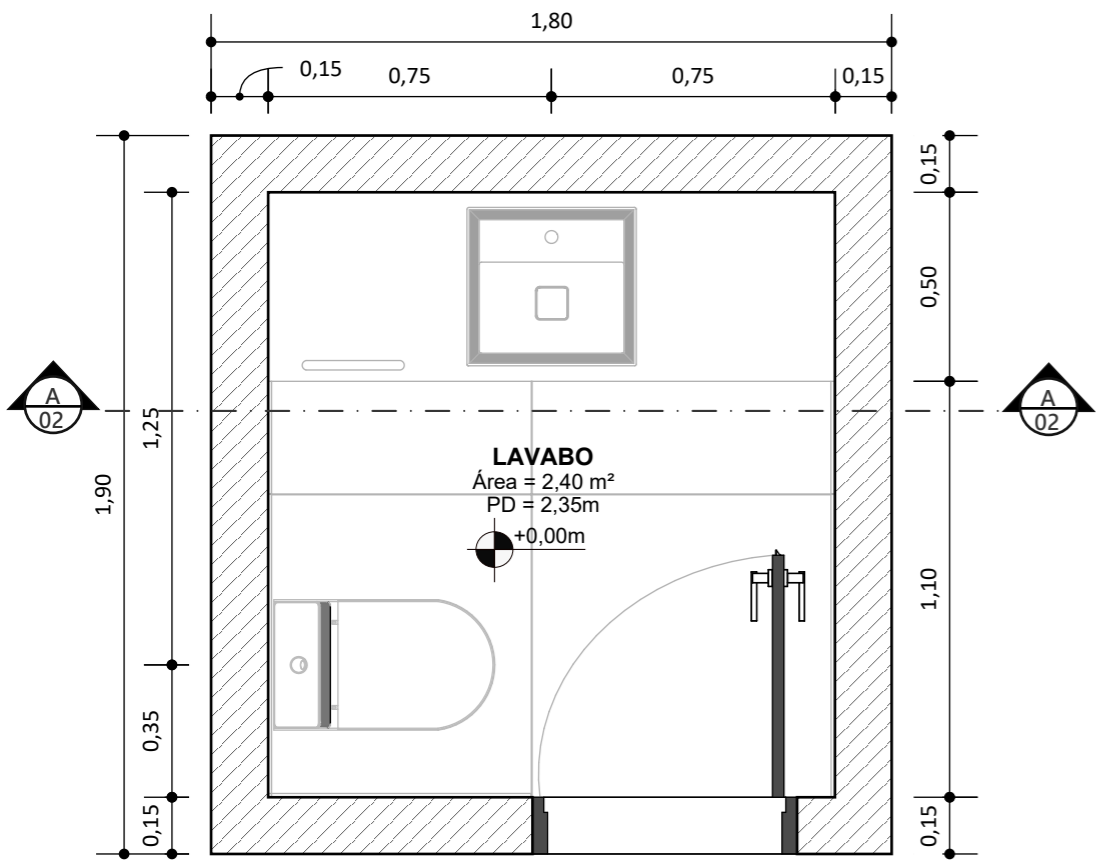
Planta Baixa - Lavabo
