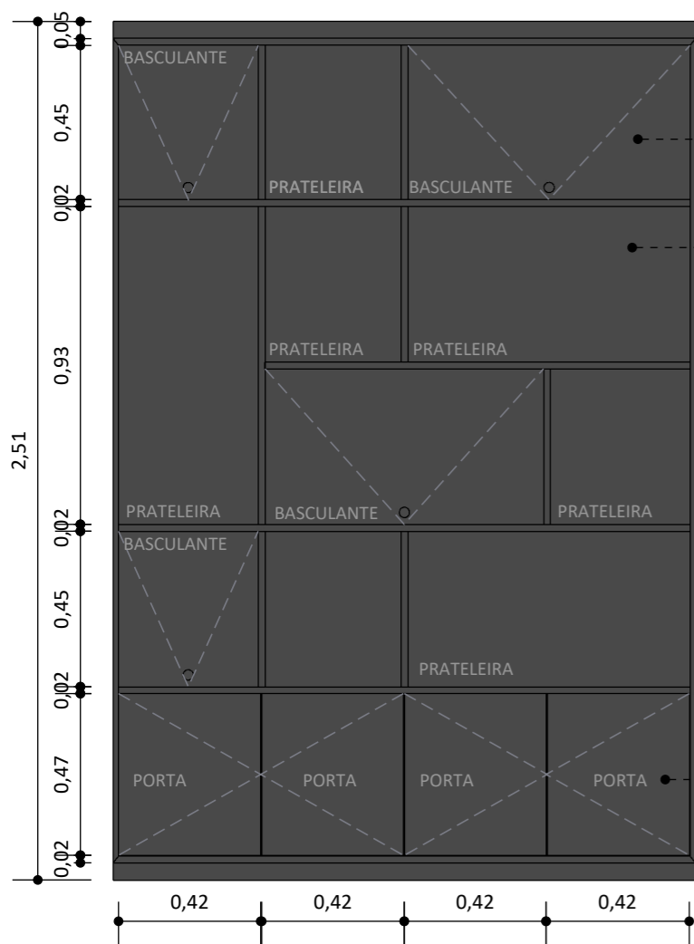
Vista Frontal - Estante
