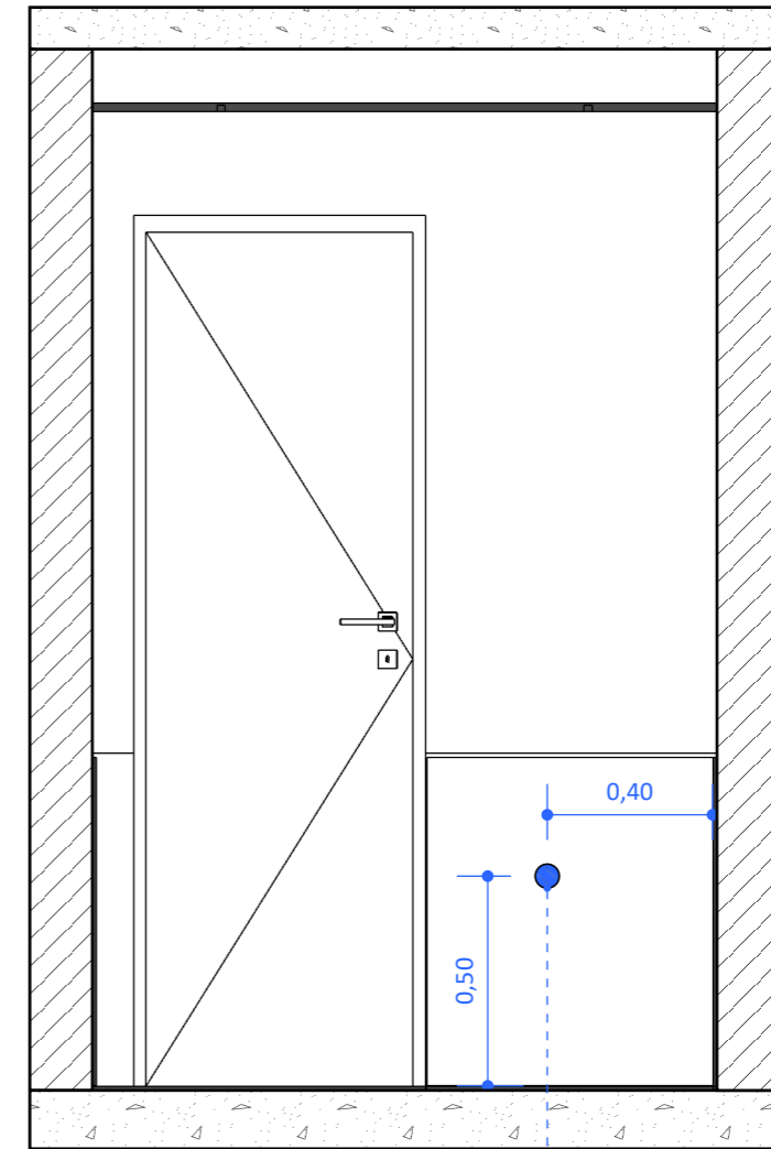
Vista C
