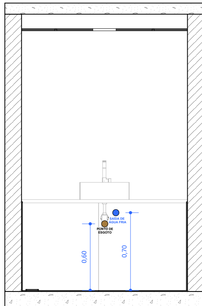
Vista A
