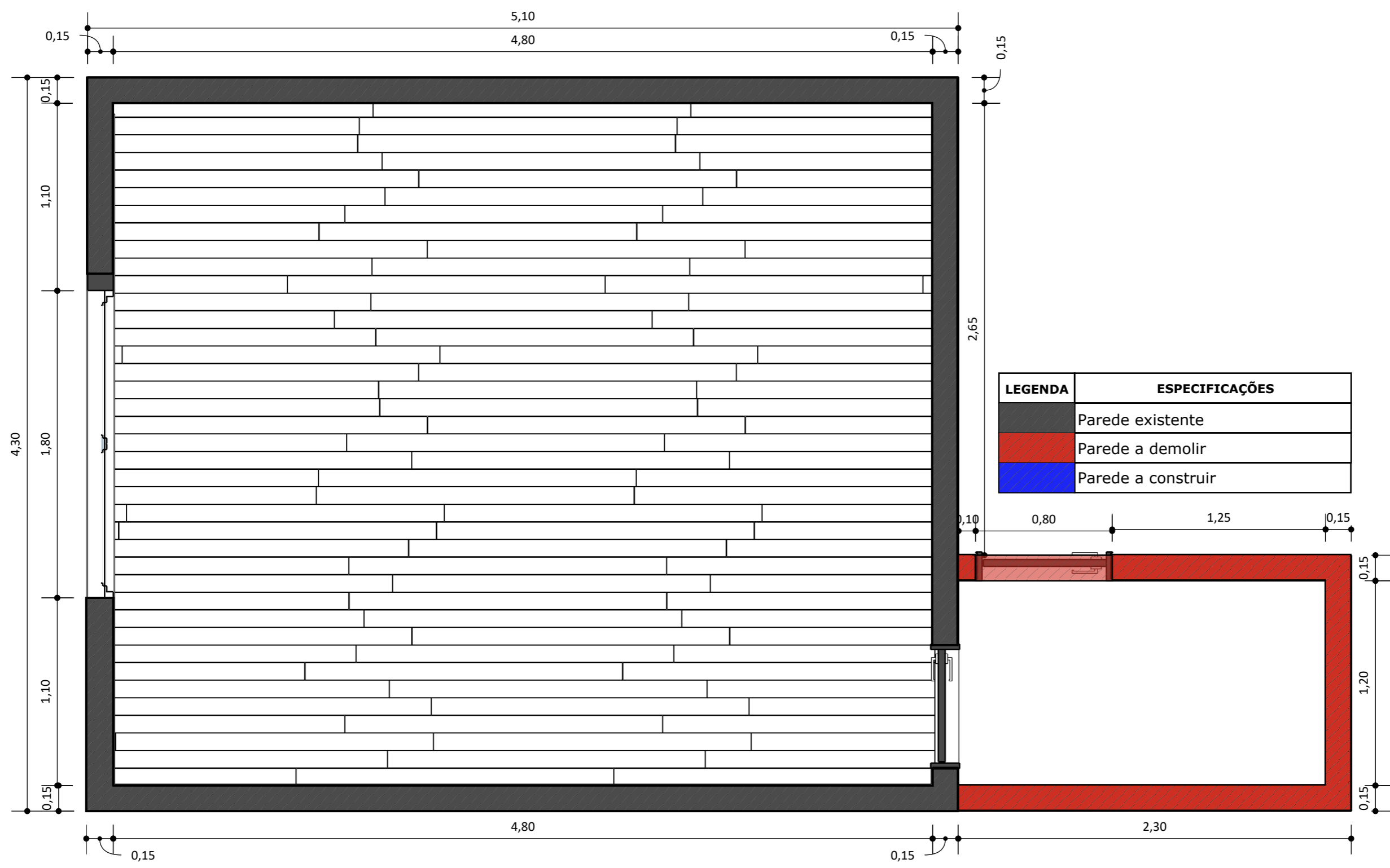
Planta de demolição
