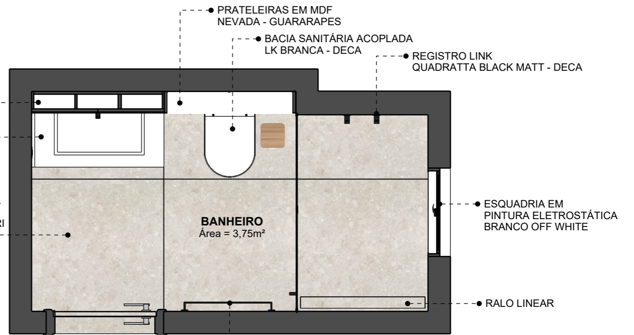
Planta de Layout Humanizada - Banheiro
