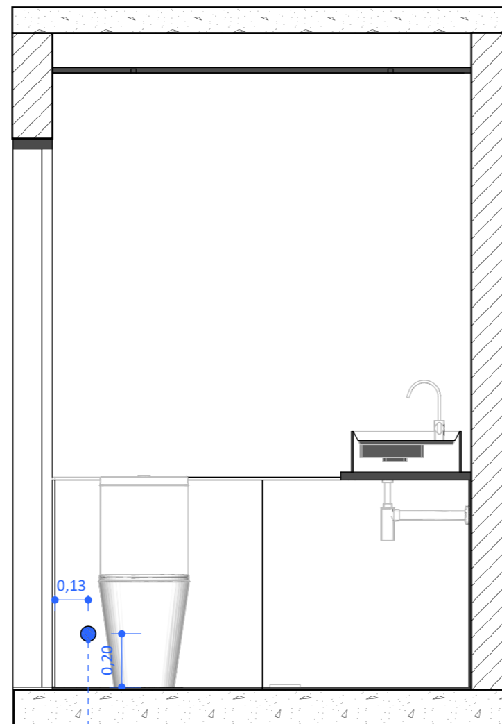
Vista B
