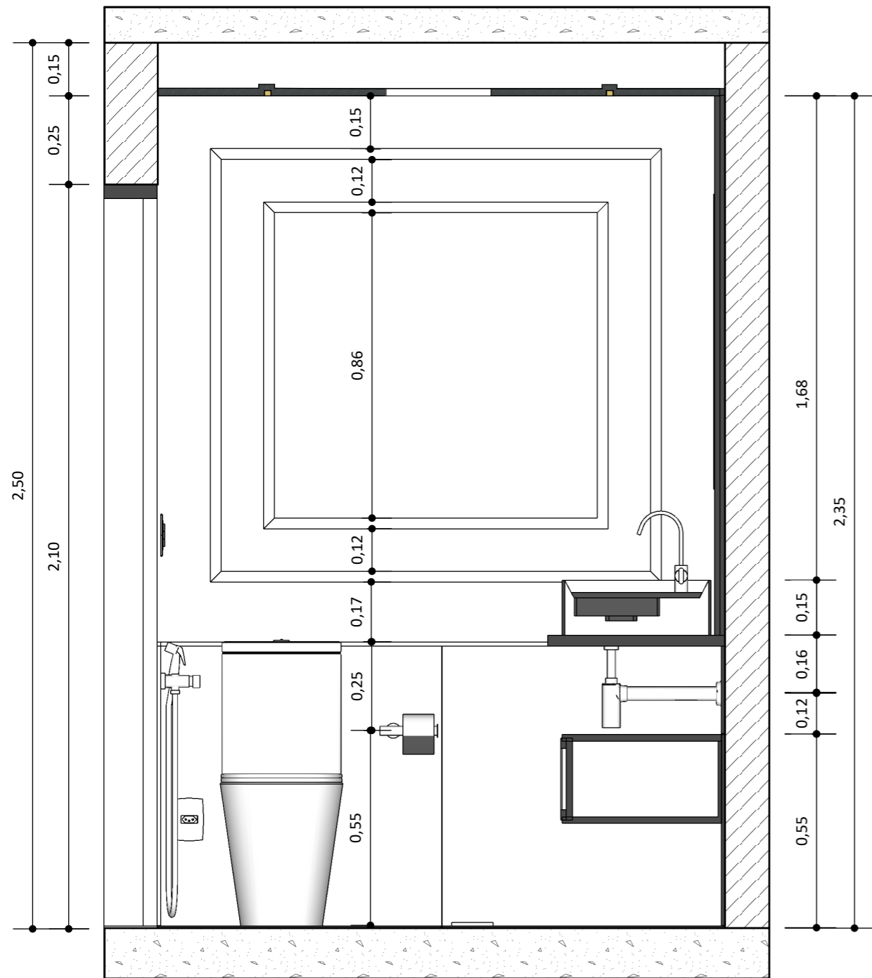
Corte B Técnico
