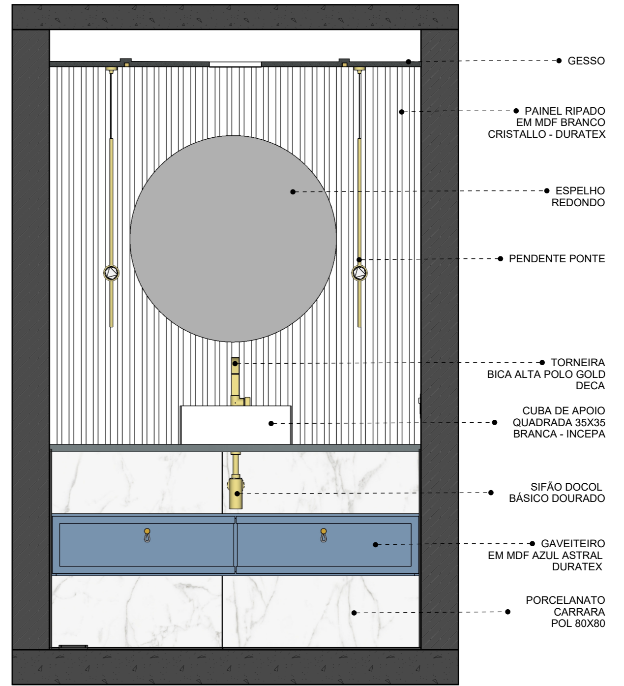
Vista A Humanizada
