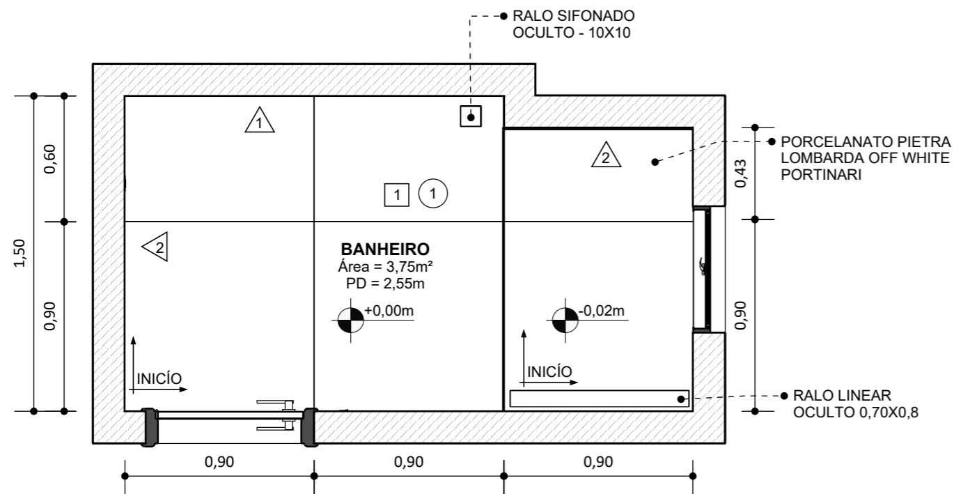
Planta de Piso
