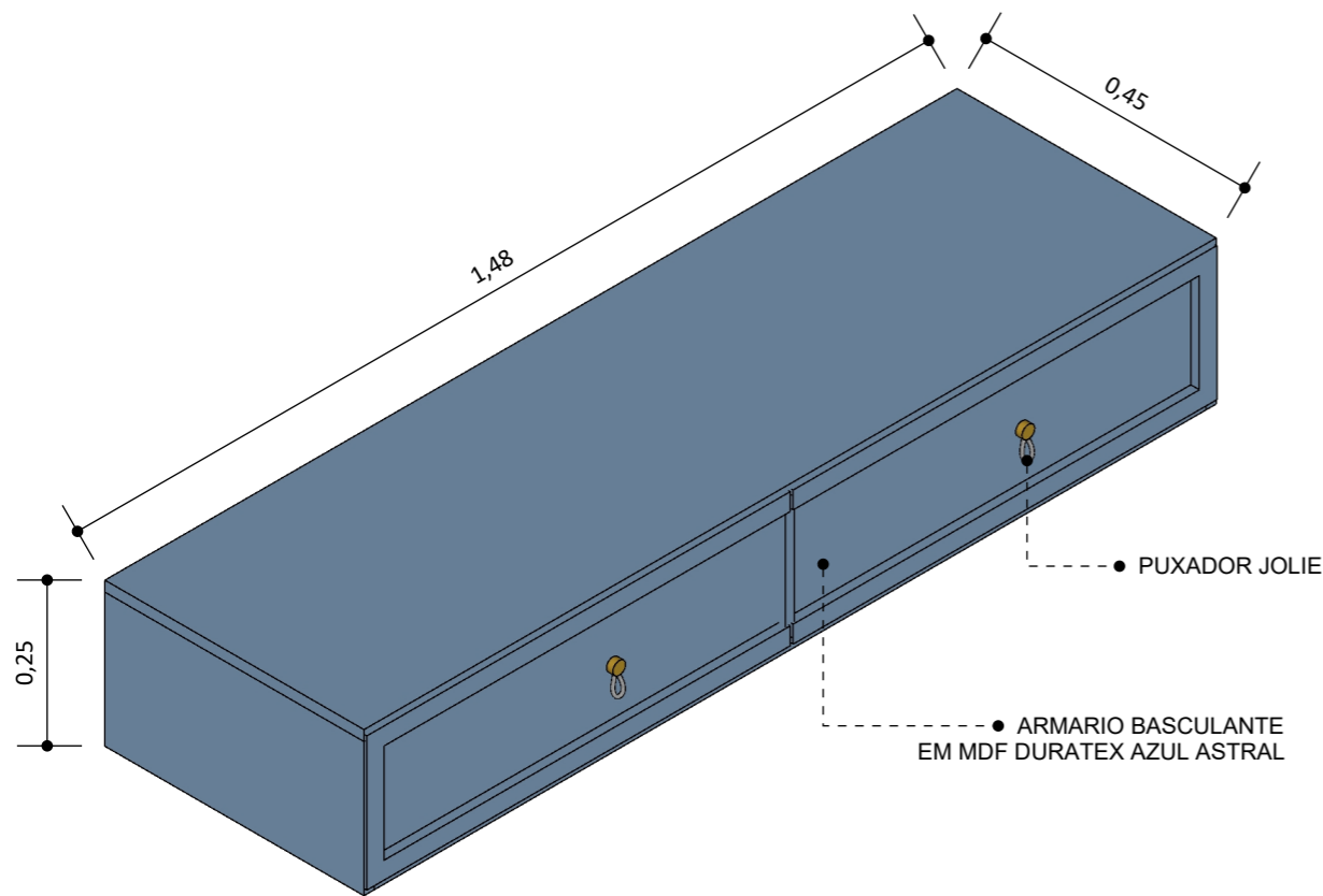
Isometrica - Armario
