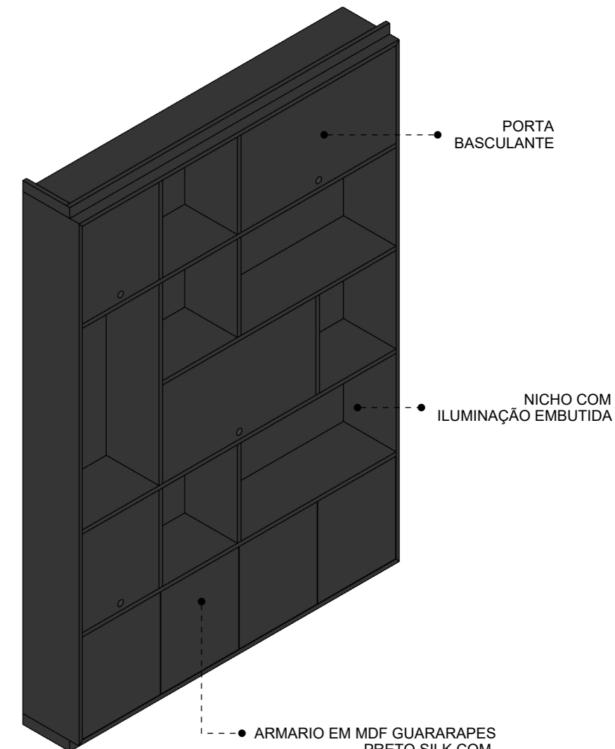
Isométrica - Estante
