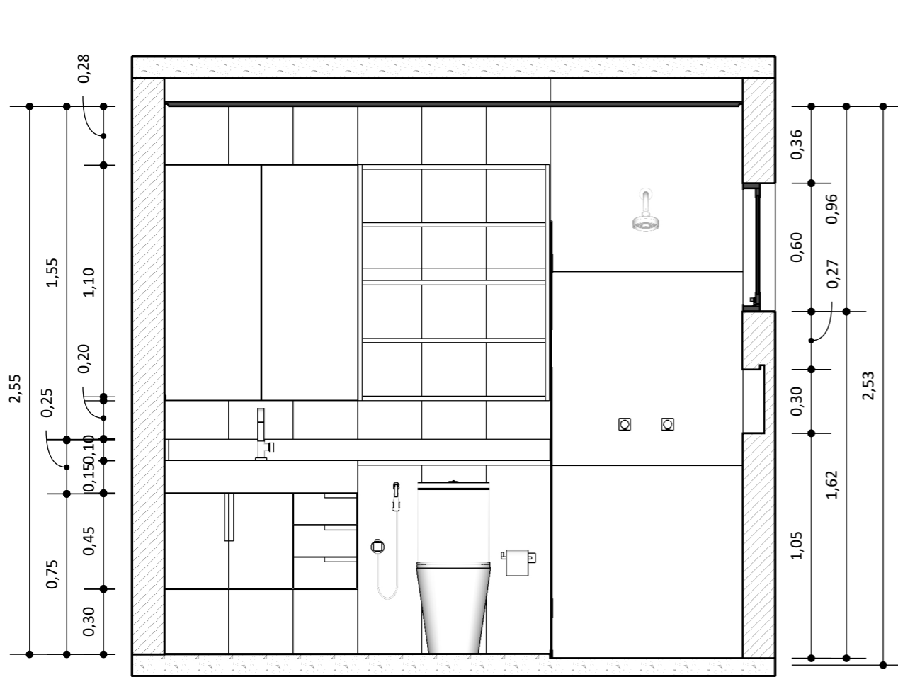
Corte A - Banheiro
