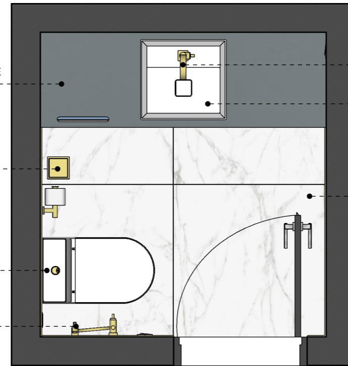
Planta de Layout
