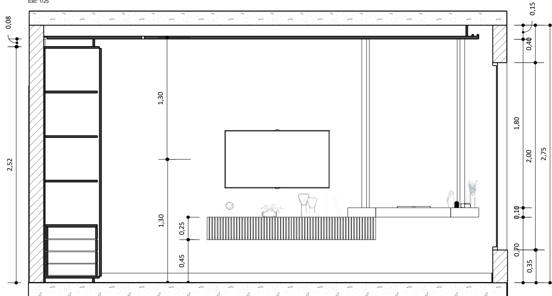
Corte D Técnico
