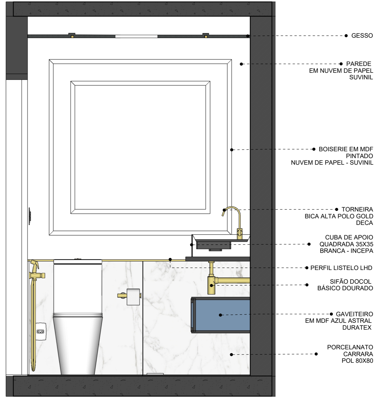
Vista B Humanizada
