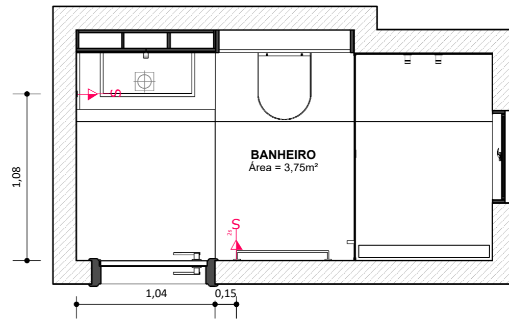
Planta de Pontos Elétricos
