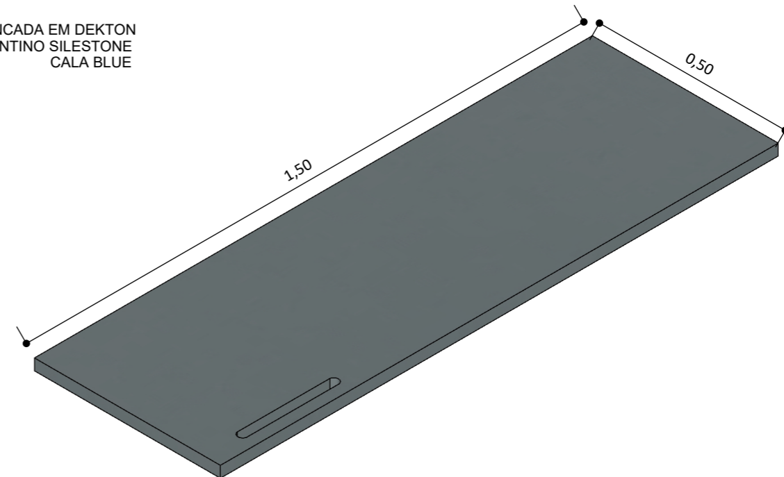
Isométrica
