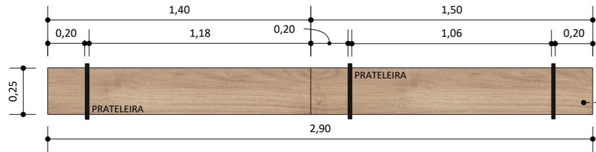
Planta Baixa - Prateleira suspensa
