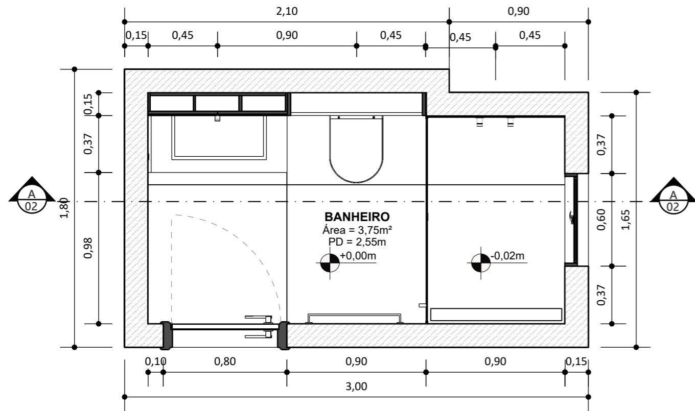
Planta Baixa - Banheiro
