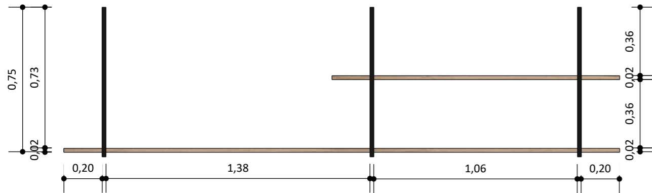
Vista Frontal - Prateleira Suspensa
