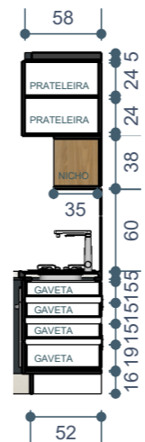
CORTE LATERAL DIREITA ESC: 1:50
