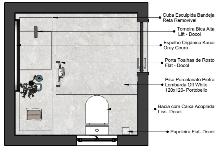
1 PLANTA BAIXA HUMANIZADA SEM ESCALA
