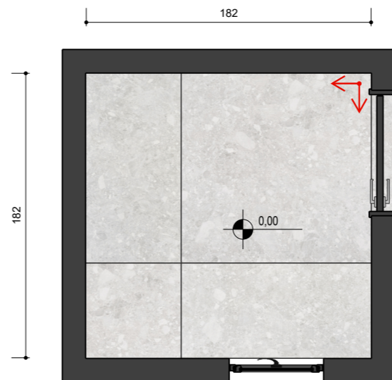
13 PLANTA PAGINAÇÃO DE PISO SEM ESCALA
