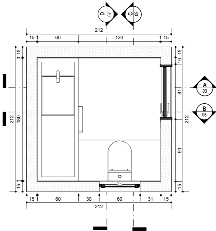
2 PLANTA BAIXA TÉCNICA SEM ESCALA
