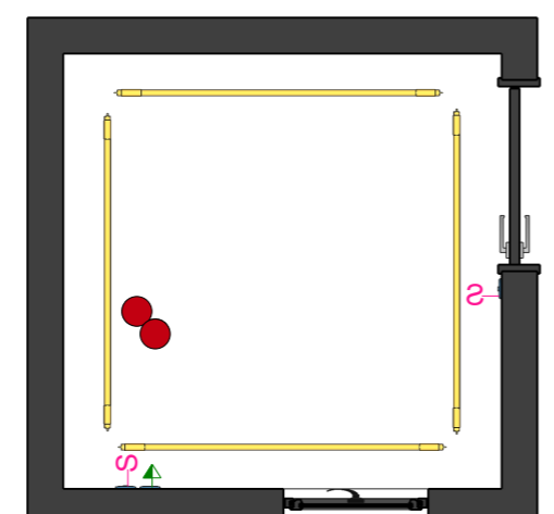
12 PLANTA LUMINOTÉCNICA E DE PONTOS ELÉTRICOS SEM ESCALA
