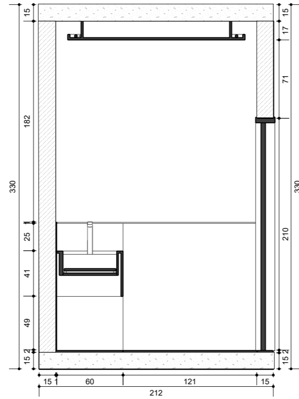
4 CORTE A TÉCNICO SEM ESCALA
