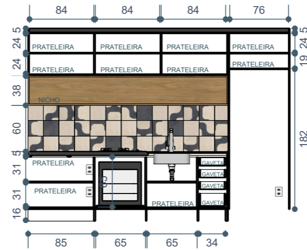
CORTE FRONTAL ESC: 1:50
