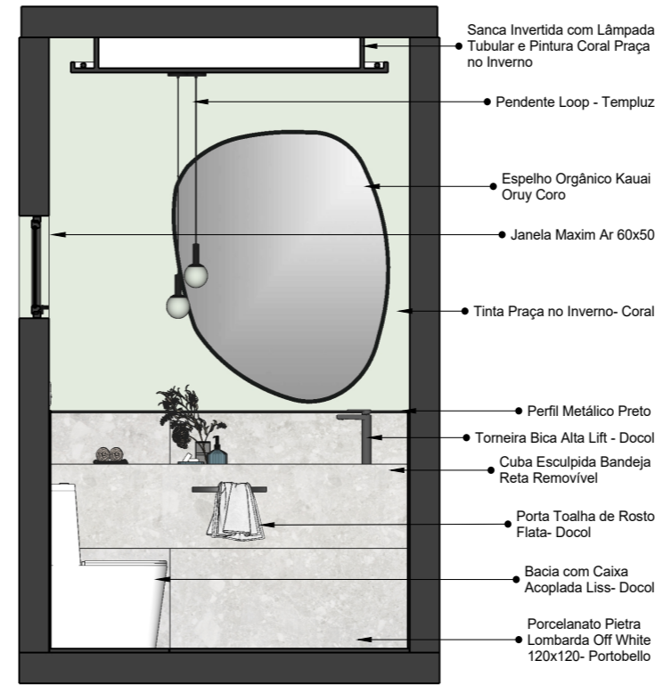
7 CORTE C HUMANIZADO SEM ESCALA
