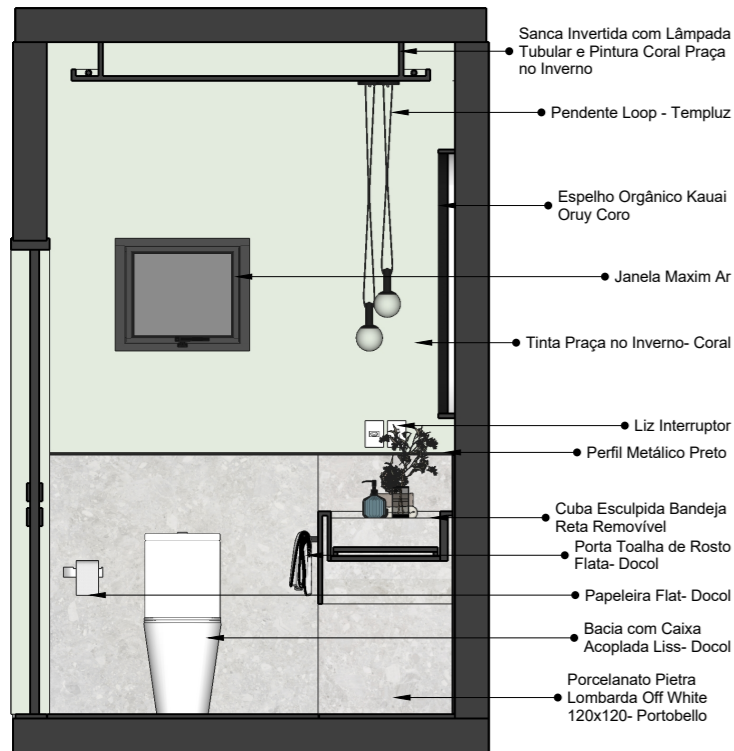
3 CORTE A HUMANIZADO SEM ESCALA
