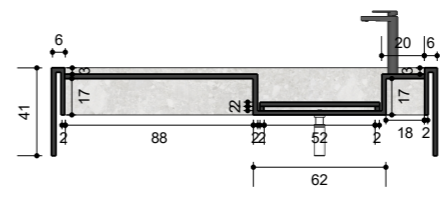
17 CORTE B SEM ESCALA
