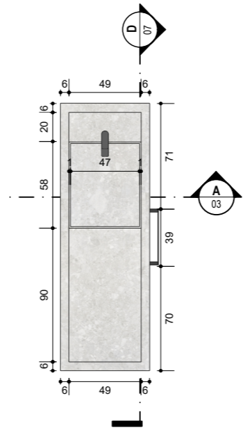
15 PLANTA CUBA ESCULPIDA SEM ESCALA
