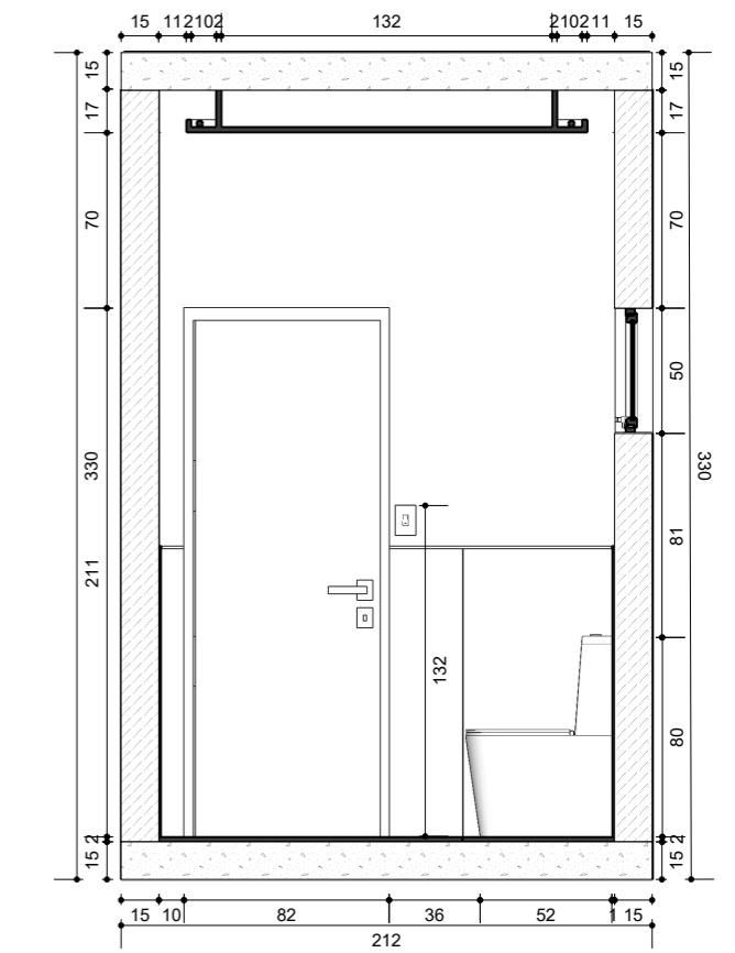
10 CORTE D TÉCNICO SEM ESCALA
