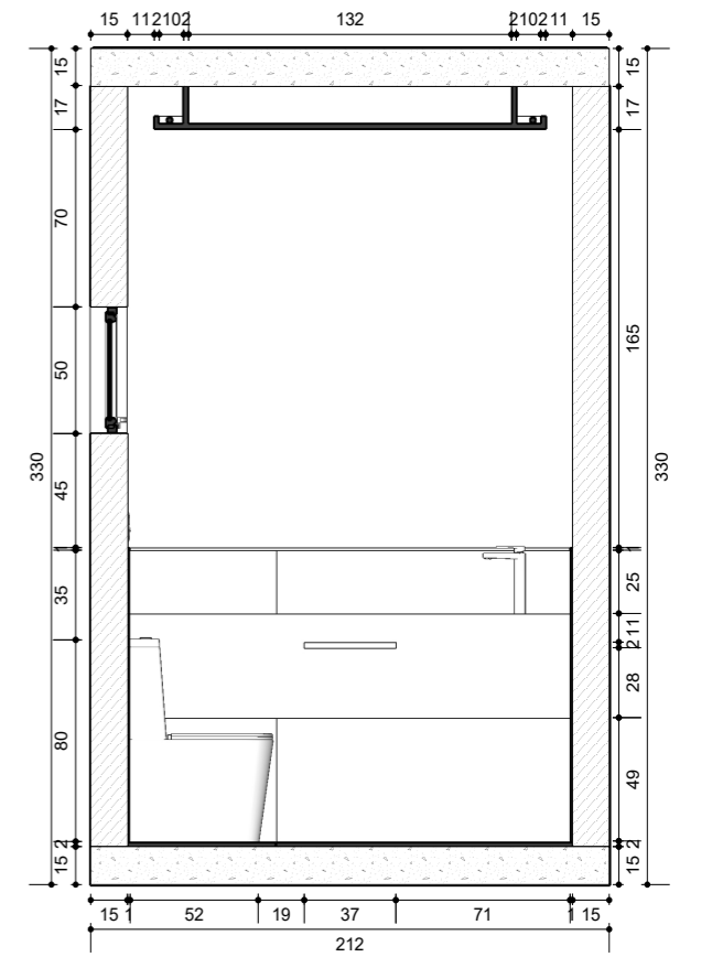
8 CORTE C TÉCNICO SEM ESCALA
