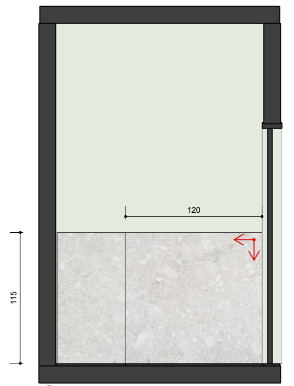
14 PLANTA PAGINAÇÃO DE PAREDE SEM ESCALA
