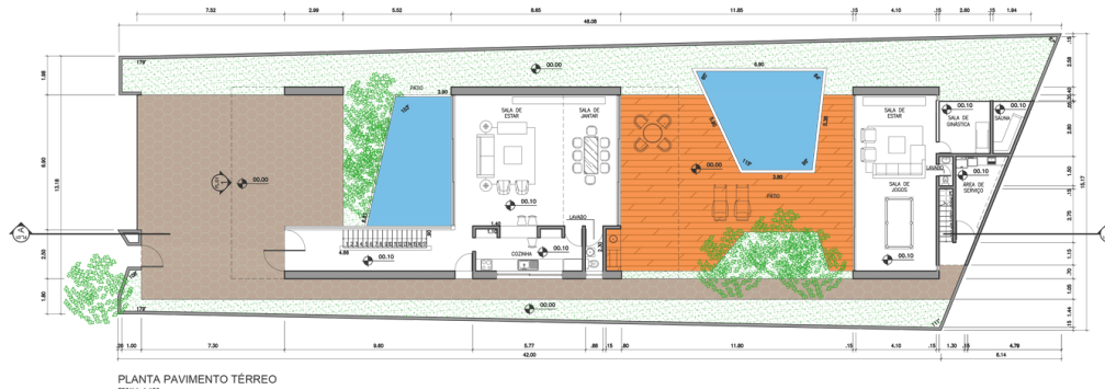
PLANTA PAVIMENTO TERREO
