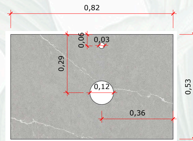
VISTA SUPERIOR BANCADA LAVABO ESCALA 1.:10
