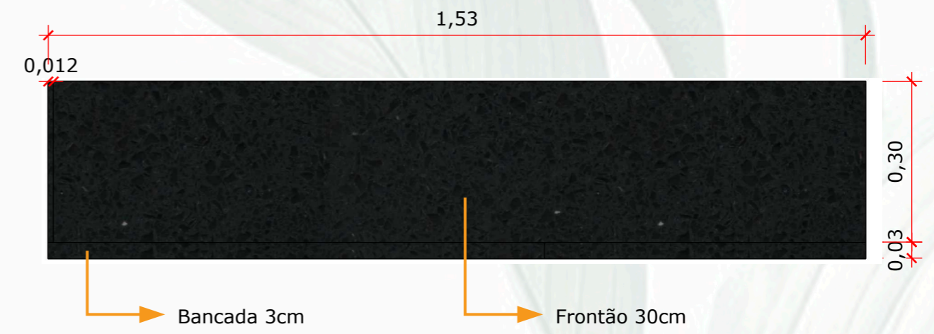
VISTA FRONTAL BANCADA/FRONTÃO ESCALA 1.:10
