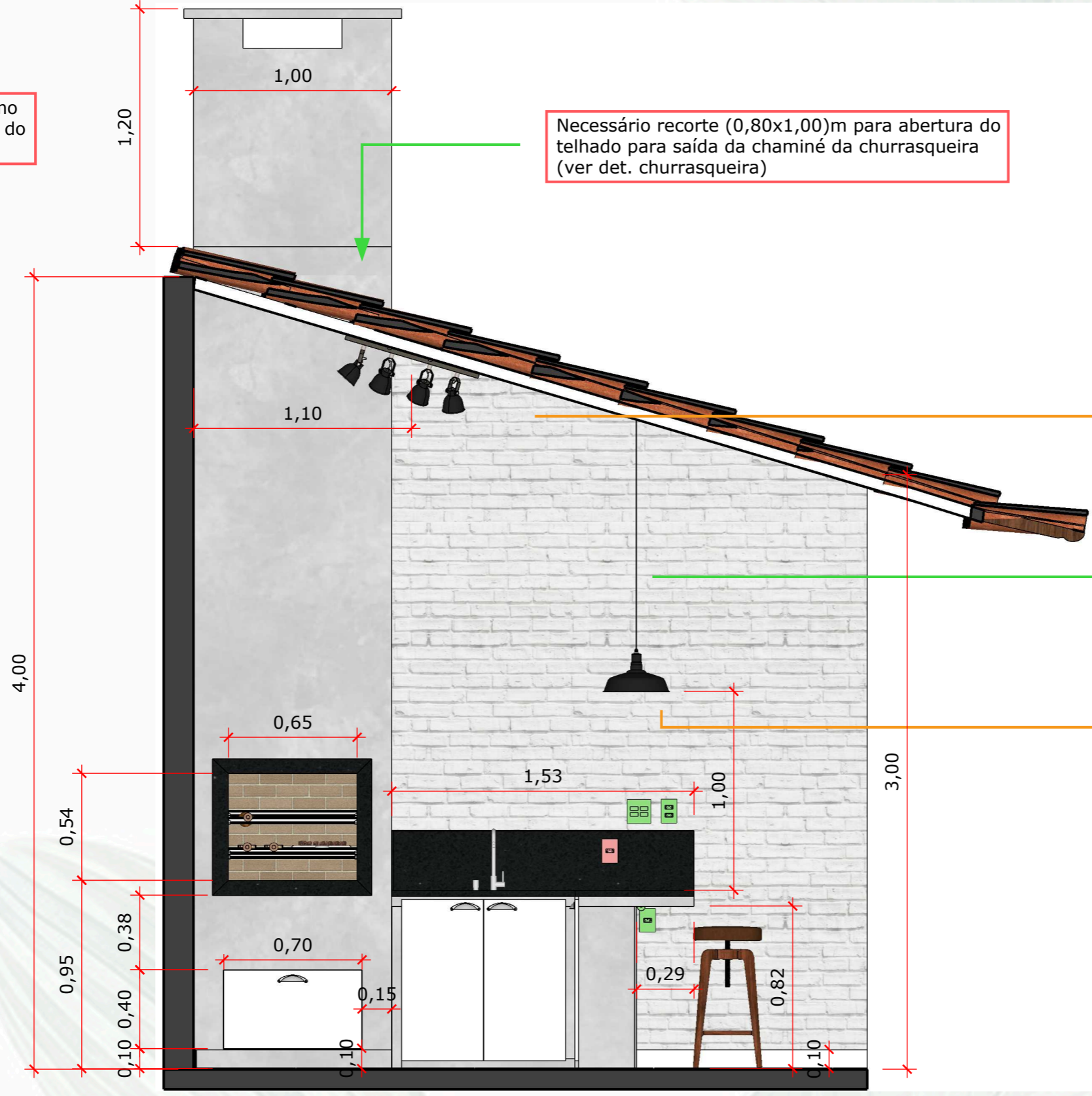
VISTA GERAL - B ESCALA 1.:25
