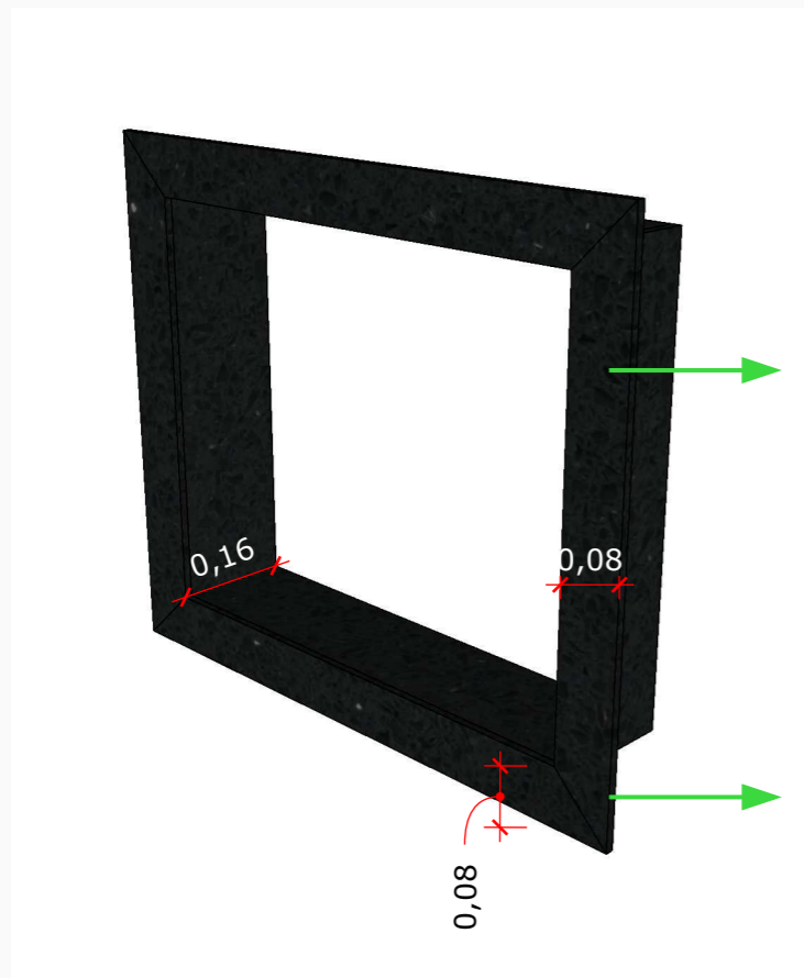
PERSPECTIVA SOLEIRA CHURRASQUEIRA SEM ESCALA
