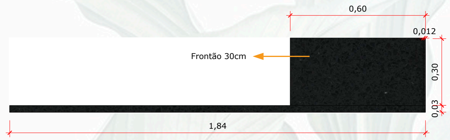
VISTA LATERAL DIREITA BANCADA/FRONTÃO ESCALA 1.:10
