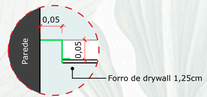
DETALHE FORRO DRYWALL LAVABO ESCALA 1.:5
