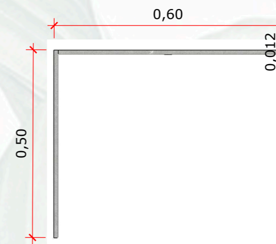
VISTA SUPERIOR FRONTÃO TANQUE ESCALA 1.:10
