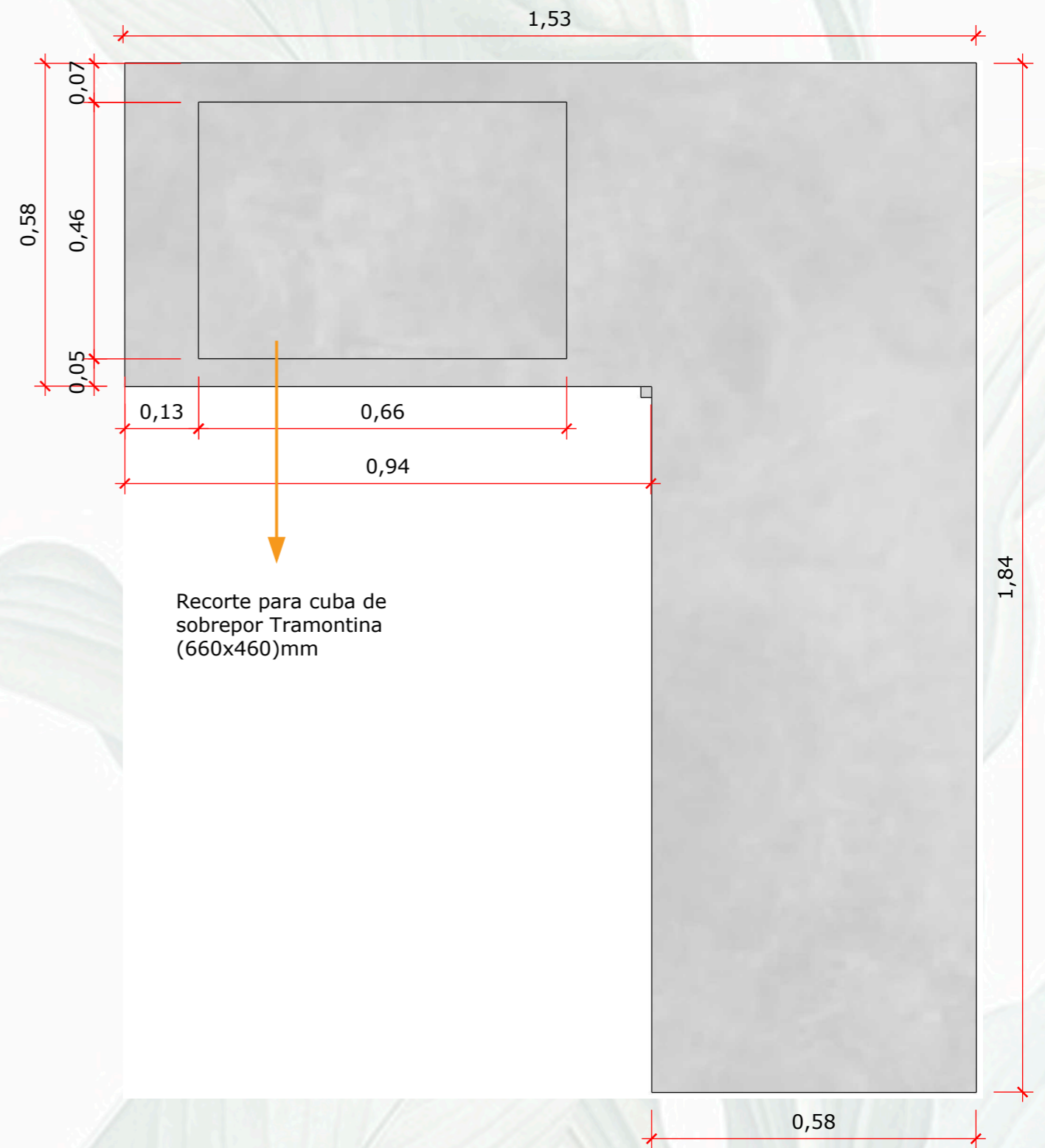
VISTA SUPERIOR BANCADA ALVENARIA ESCALA 1.:10
