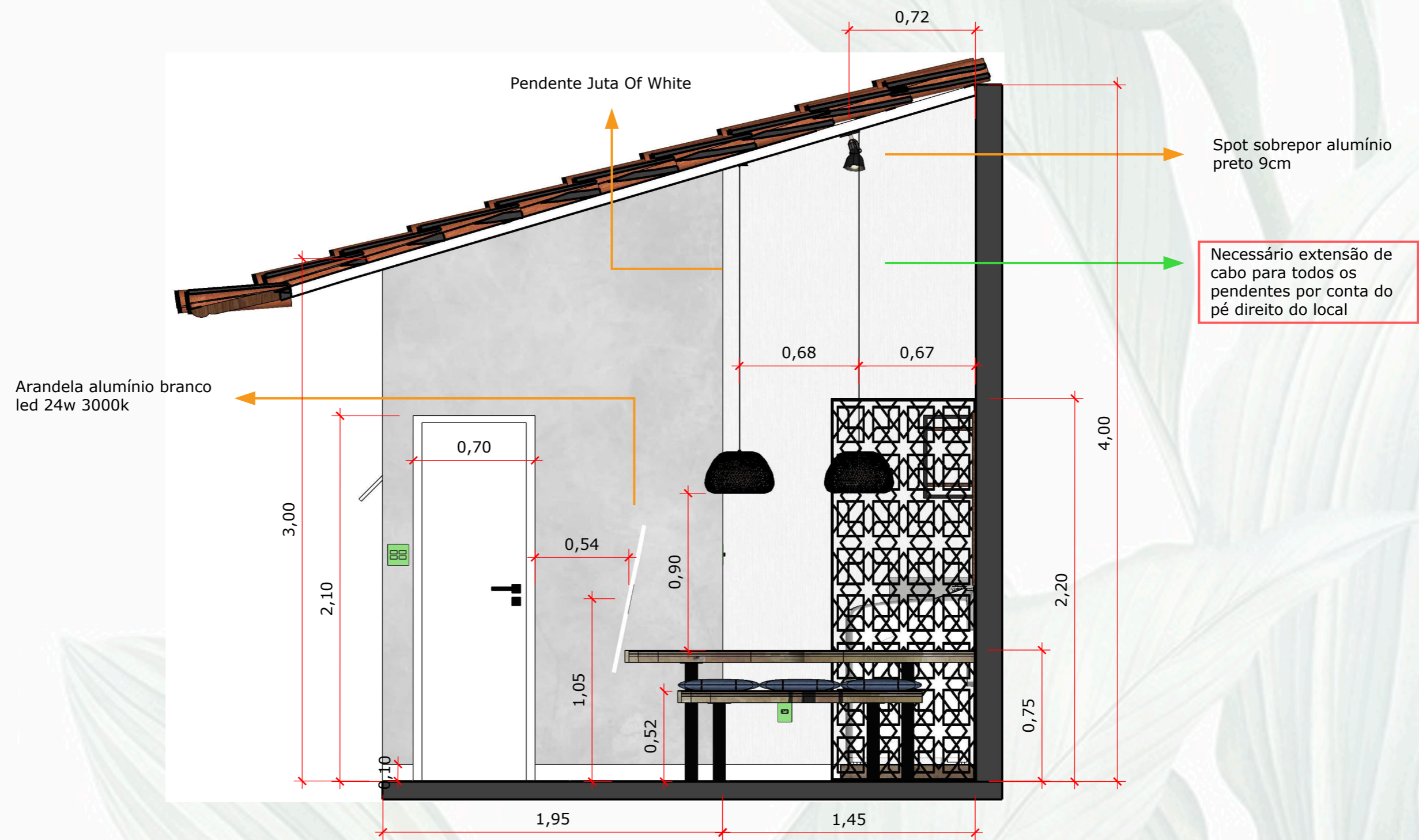
VISTA GERAL - C ESCALA 1.:25
