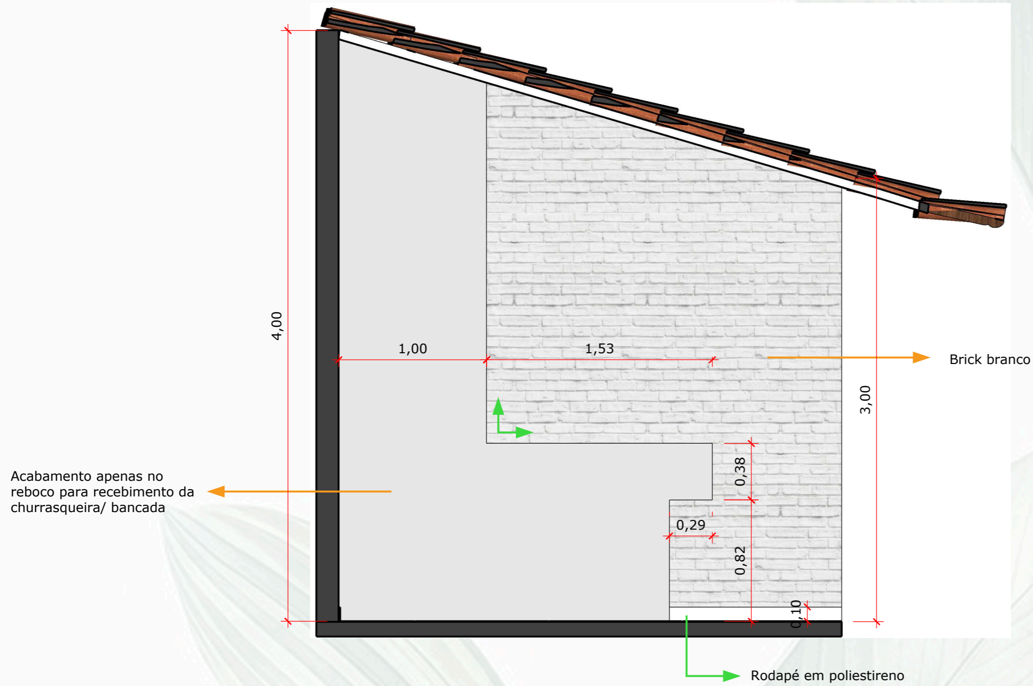
VISTA REVESTIMENTOS - B ESCALA 1.:25
