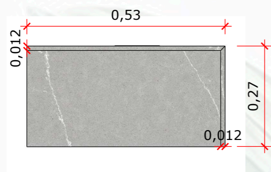
VISTA LATERAL ESQUERDA BANCADA LAVABO ESCALA 1.:10
