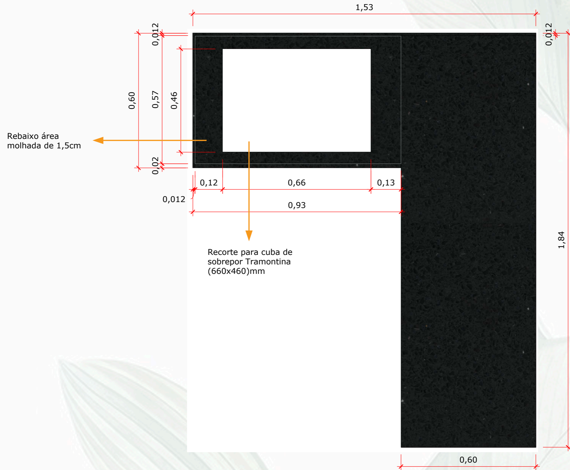
VISTA SUPERIOR BANCADA/FRONTÃO ESCALA 1.:10
