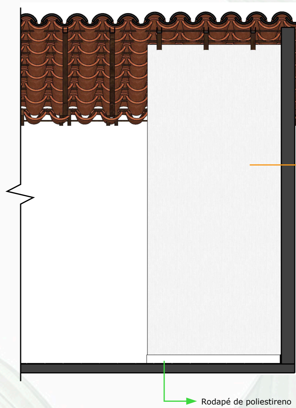
VISTA REVESTIMENTOS - E ESCALA 1.:25
