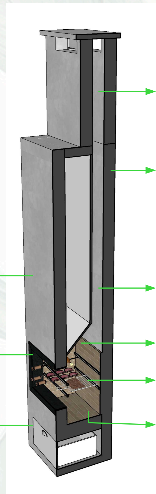
PERSPECTIVA EM CORTE CHURRASQUEIRA SEM ESCALA
