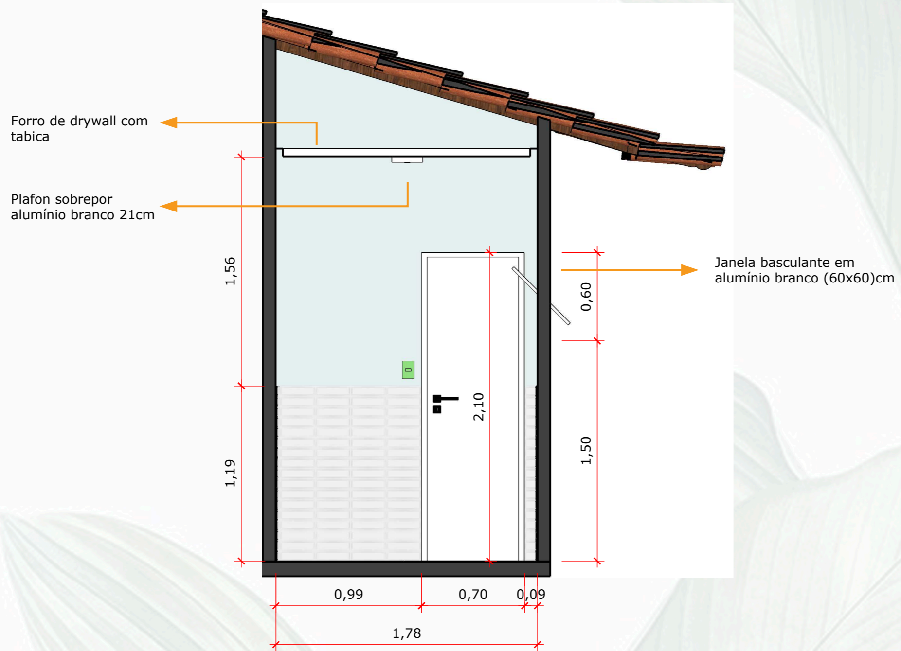
VISTA GERAL - F ESCALA 1.:25
