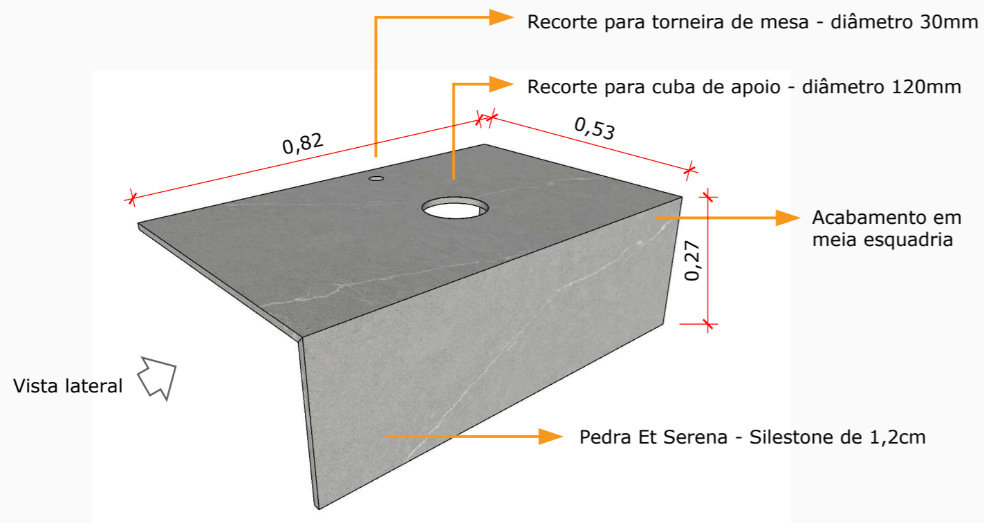
PERSPECTIVA BANCADA LAVABO SEM ESCALA
