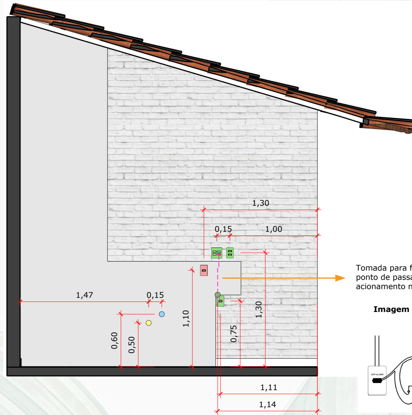
VISTA PONTOS TÉCNICOS - B ESCALA 1.:25
