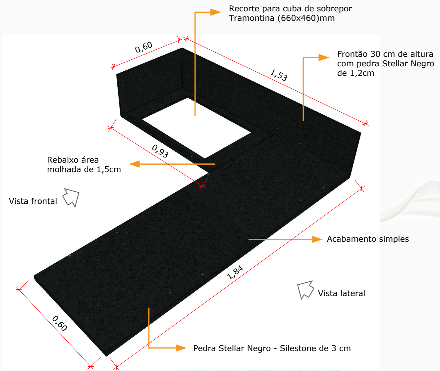
PERSPECTIVA BANCADA/FRONTÃO SEM ESCALA
