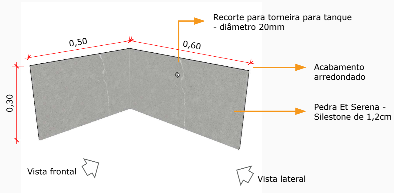
PERSPECTIVA FRONTÃO TANQUE SEM ESCALA
