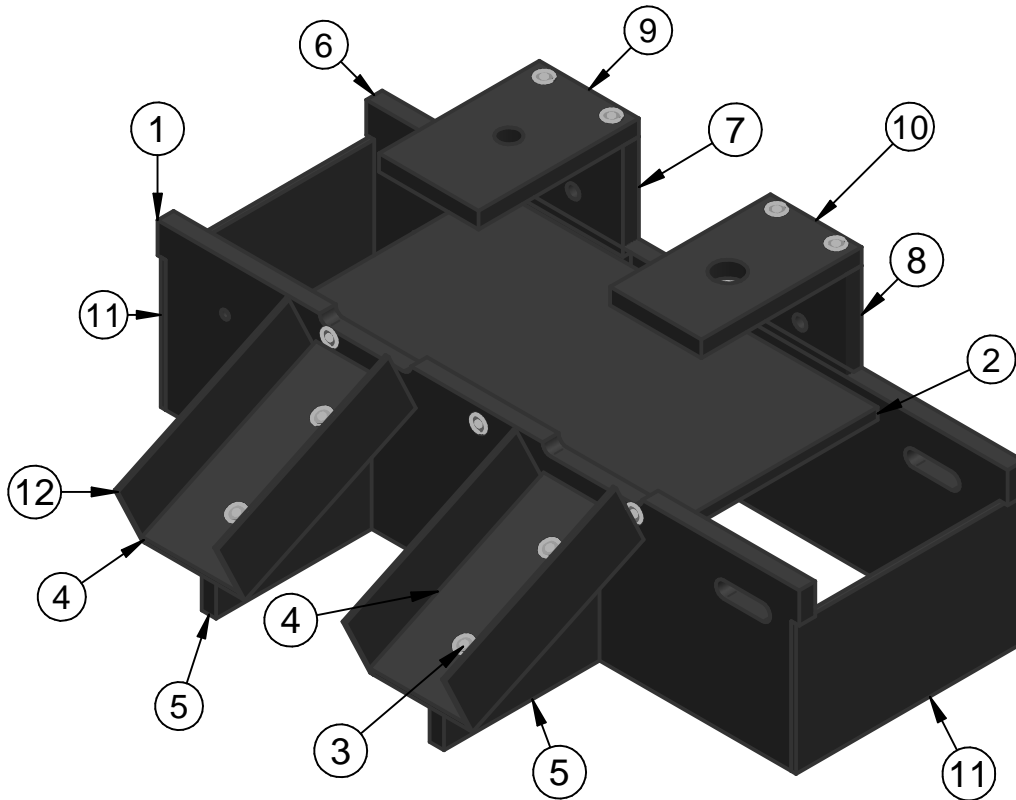
VISTA ISOMÉTRICA ESTEIRA
