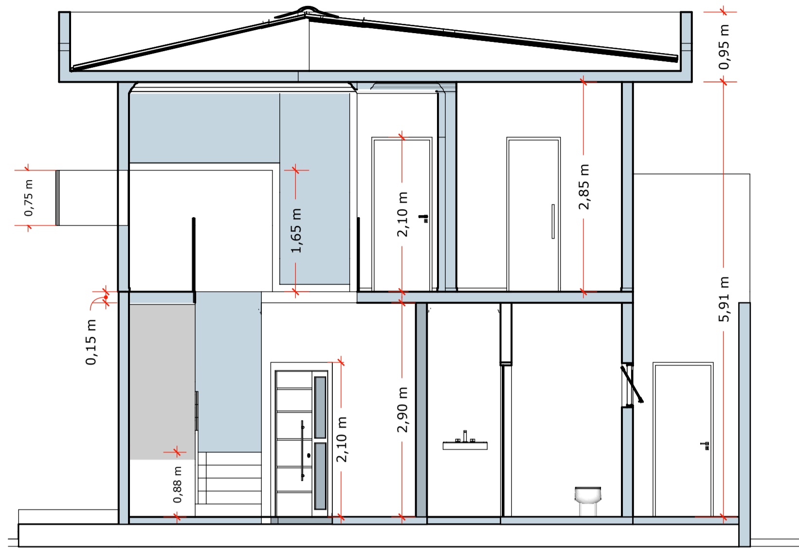
Corte A
