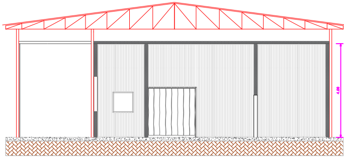
CORTE A-A
