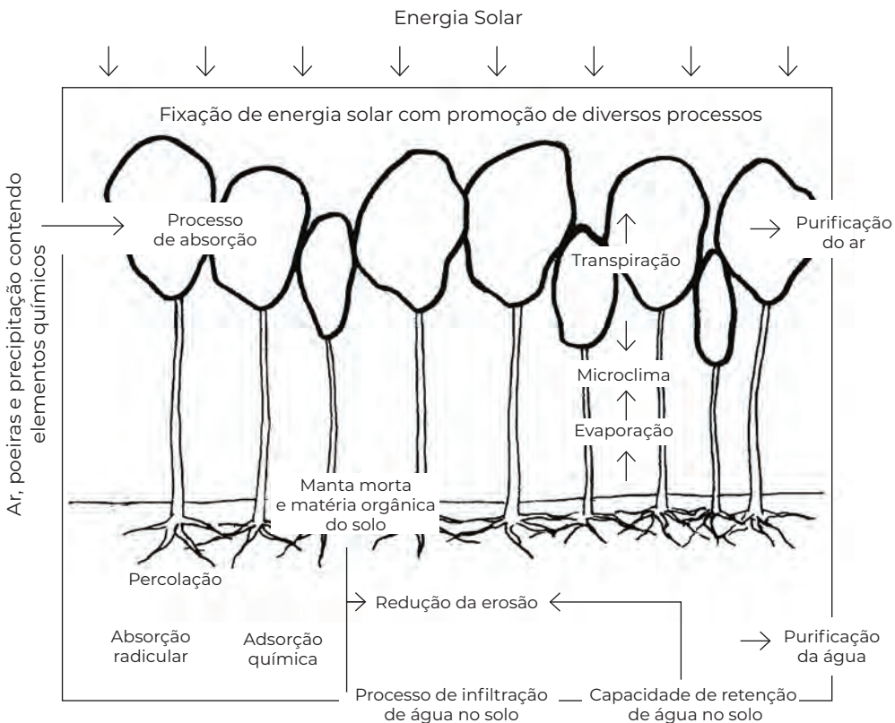
Figura 3.4 Através da regulação do fluxo de energia, como suporte de processos activos e passivos, ocorre nesta fase um controlo sobre o microclima, os ciclos energético, hidrológico, biogeoquímico e o regime de decomposição (a partir de Bormann e Likens, 1994).
