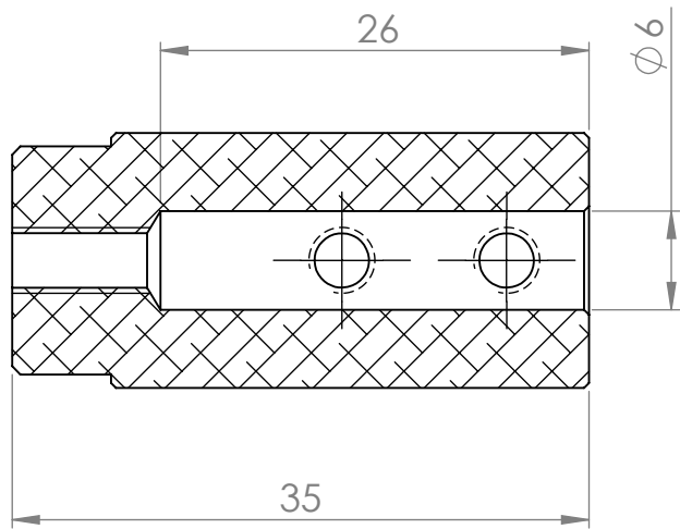
SEÇÃO B-B
