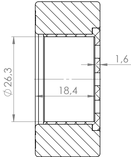
SEÇÃO AA-AA ESCALA 3 : 2
