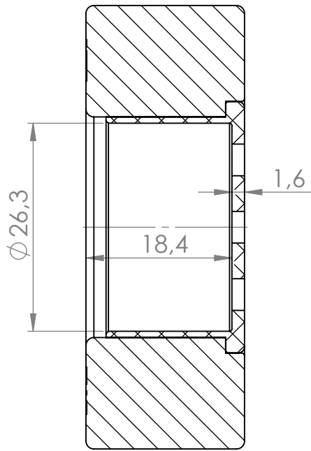
SEÇÃO AB-AB
