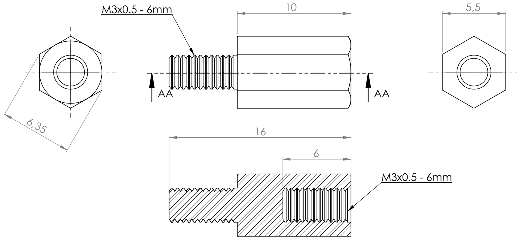
SEÇÃO AA-AA ESCALA 5 : 1
