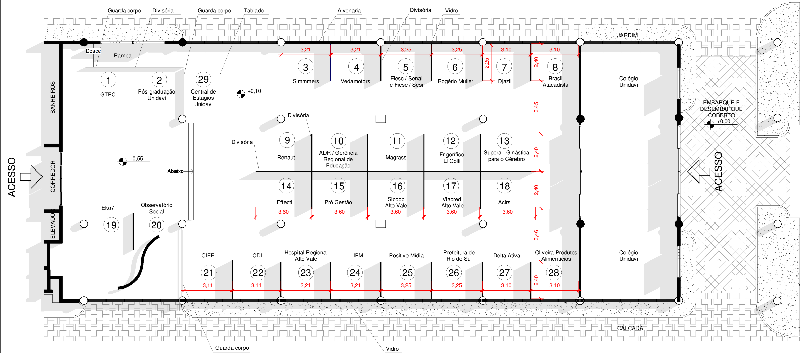
1 PLANTA BAIXA - TÉRREO 1 : 125
