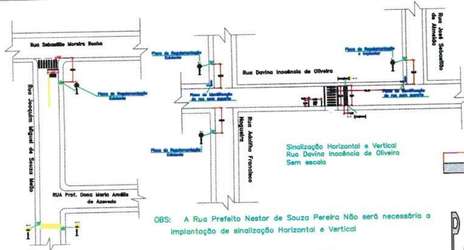
e LRE (linha de retenção) Manual Brasileiro de Sinalização de Tráfego - volume IV - páginas 38 e 108. Cor: BRANCA (N 9,5).
