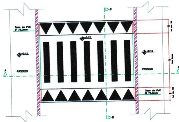
Detalhe de Faixa Elevada
