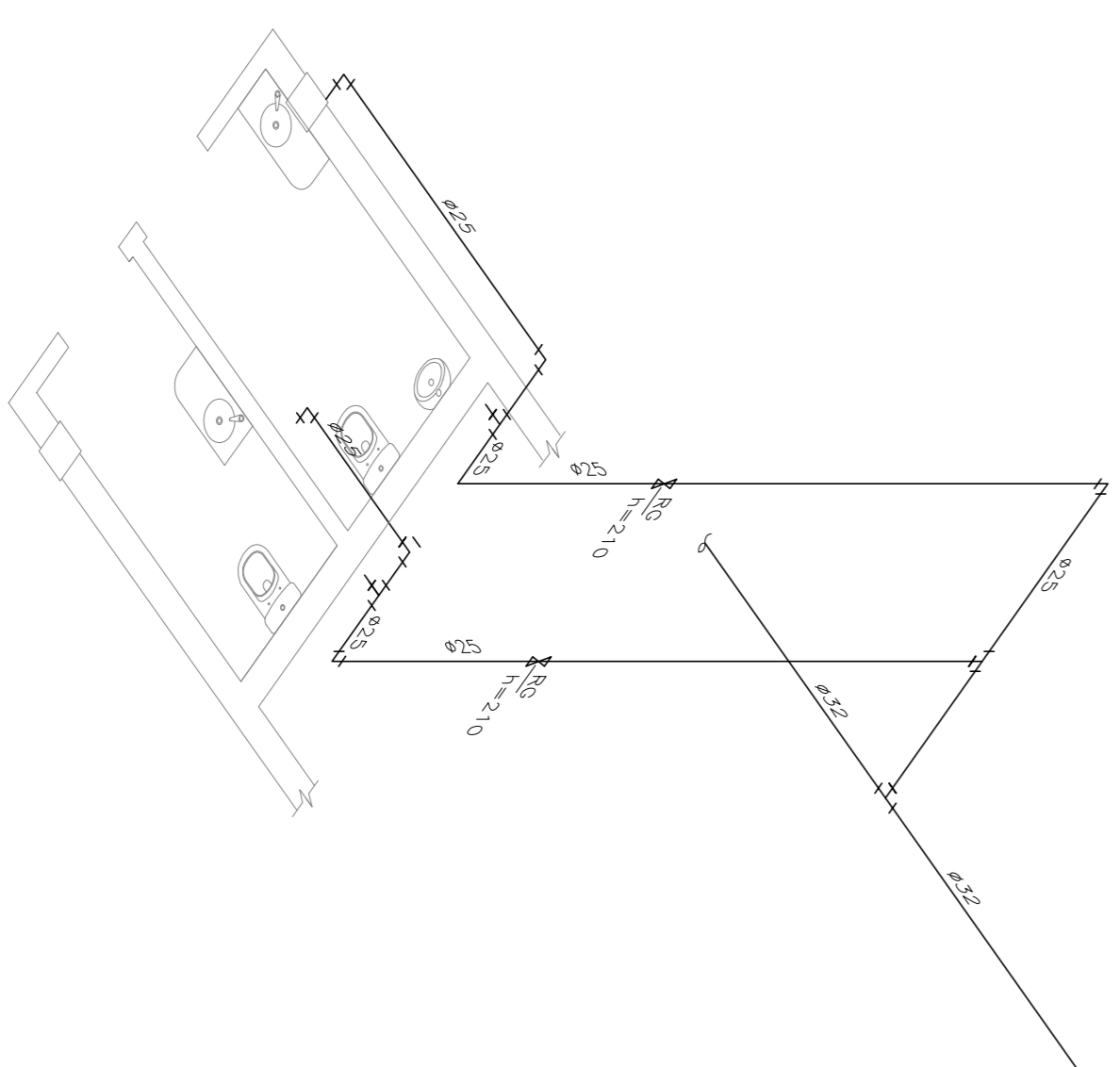
DIAGRAMA ISOMÉTRICO Esc. 1/50
